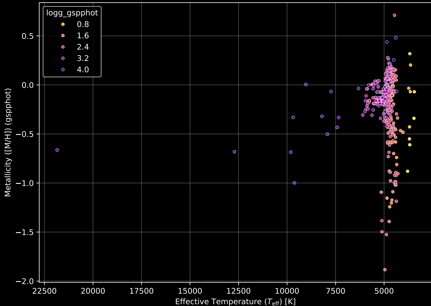
APOGEE DR17 Field: [015-12] Stellar Population Parameters (n= 355)
